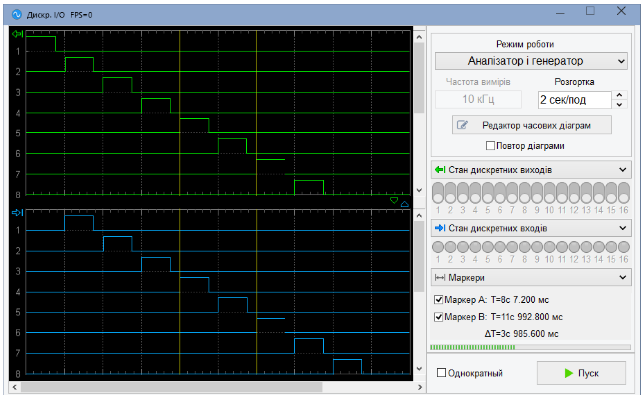
Рисунок 10.11.2.1 – Зовнішній вигляд панелі «Дискр. І/О»
