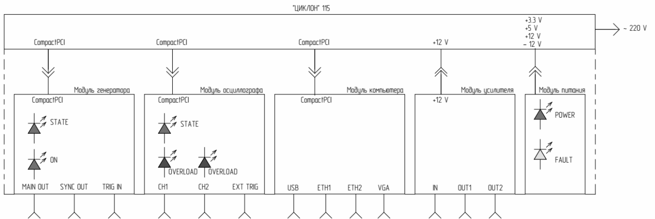
Рисунок 6.1.1 – Структура приладу
