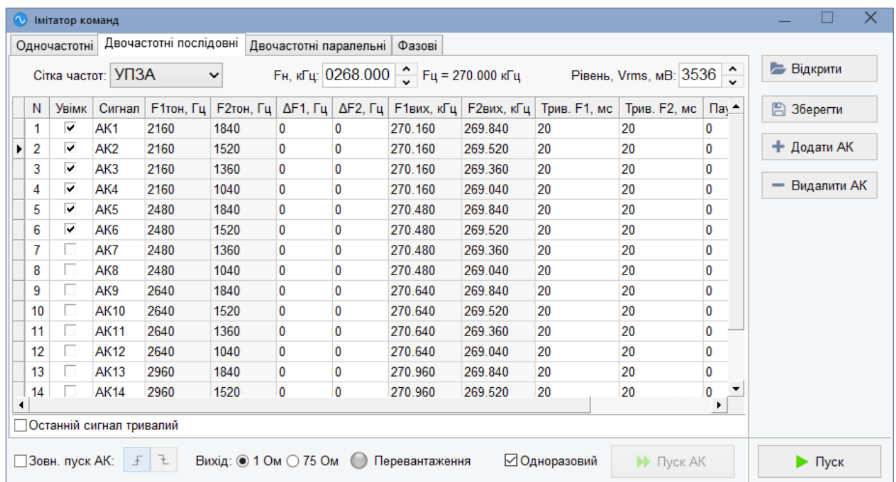
Рисунок 10.8.4.1 – Зовнішній вигляд панелі імітатора команд «Двочастотні послідовні»
