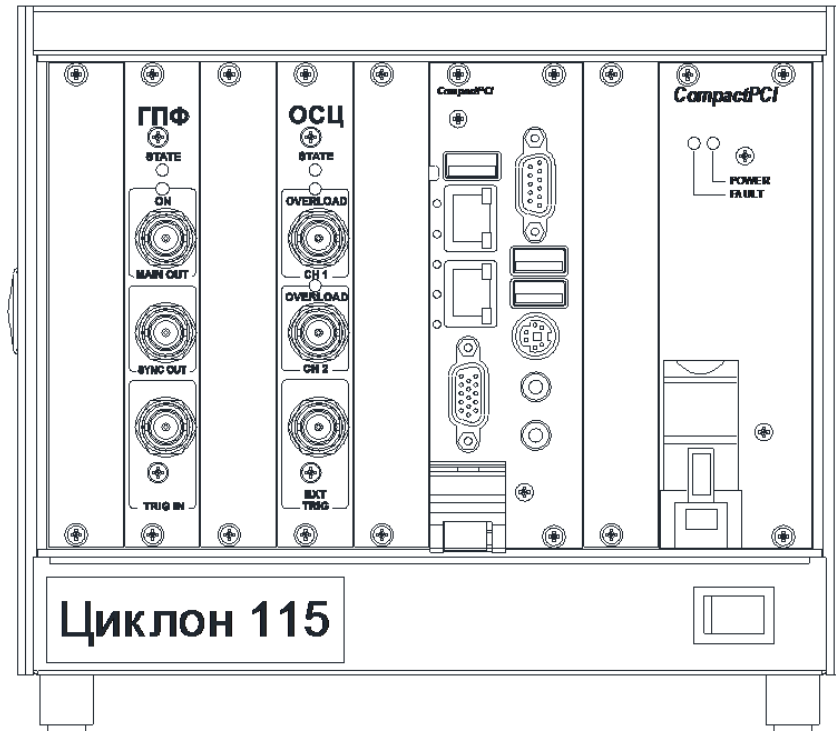
Рисунок 4.1.1 – Зовнішній вигляд приладу (Модифікація 1)
