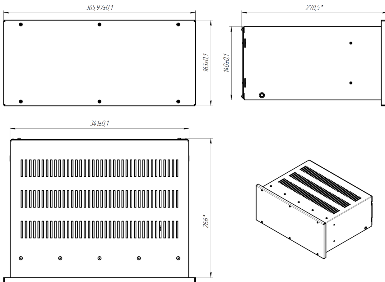
Рисунок 3.2 - Габаритні розміри (APC B)
