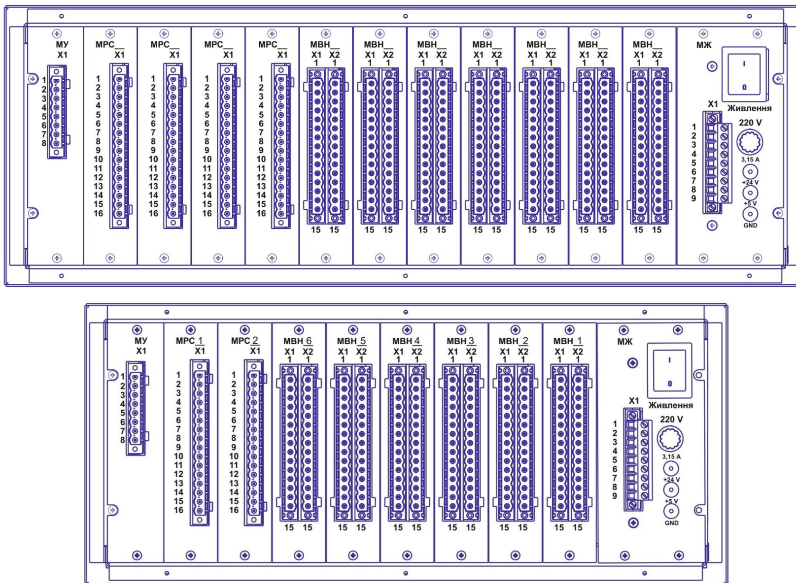
Рисунок 3.8 – Зовнішній вигляд «ОПІОН» APC (виконання APC MODBUS) зі сторони підключення
