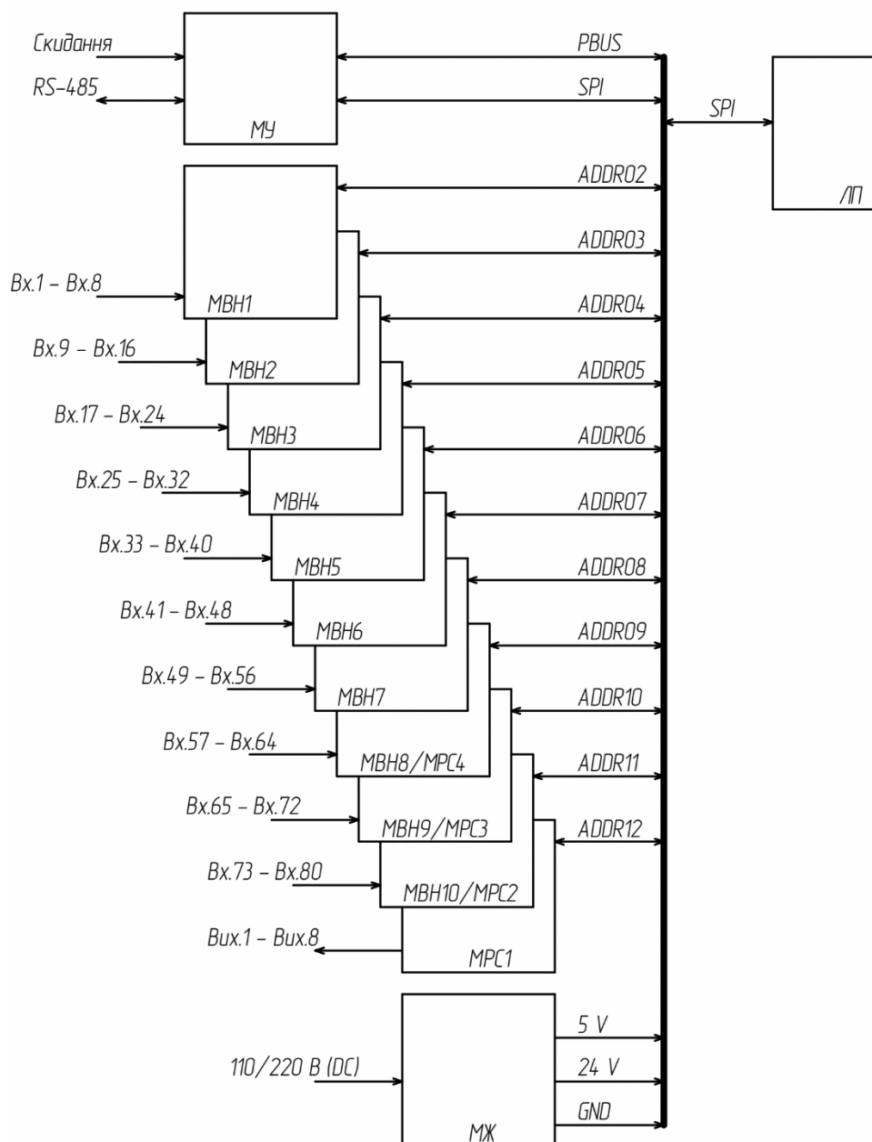
Рисунок 6.1.1 – Структурна схема APC виконання «MODBUS»
