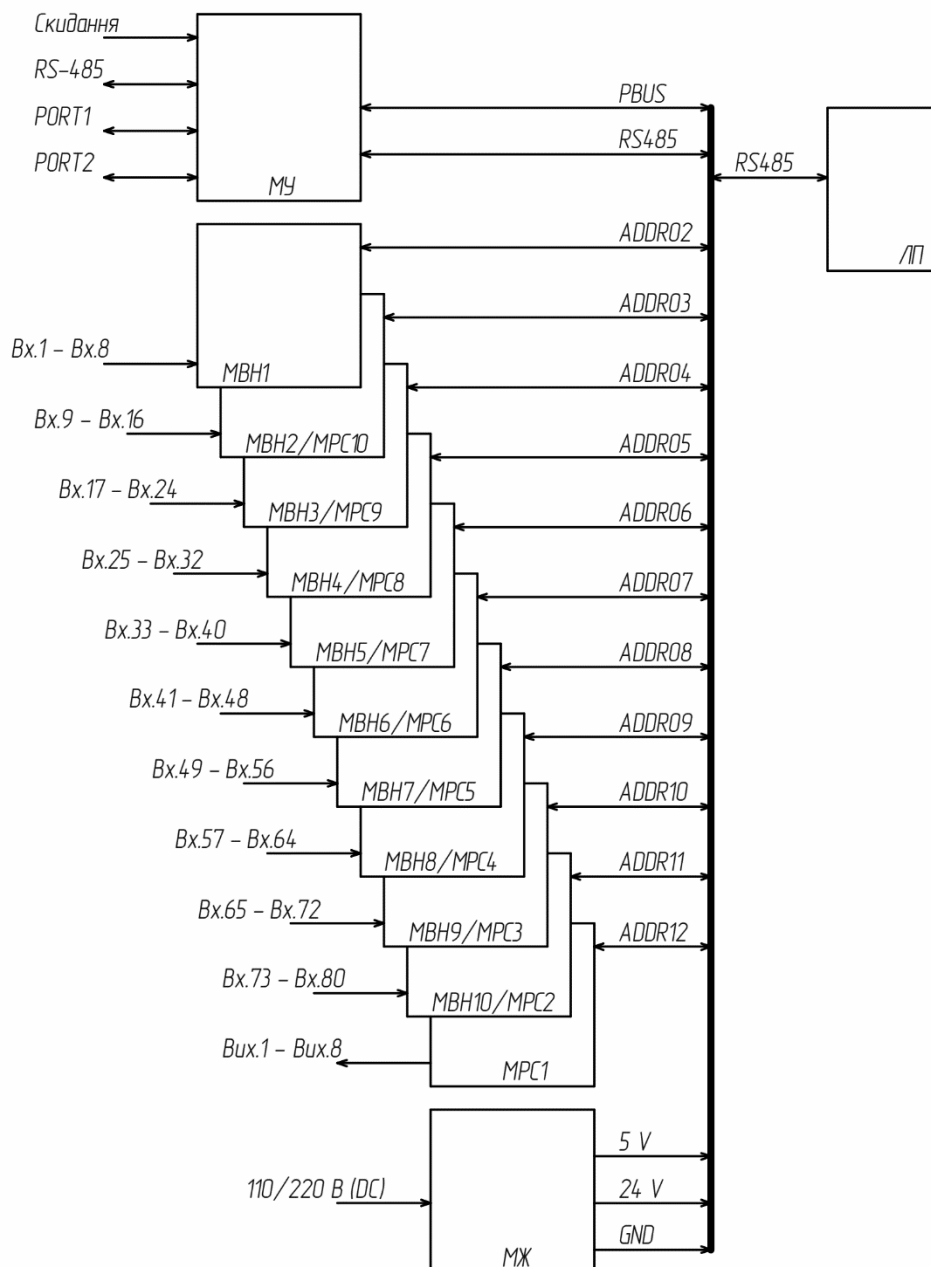
Рисунок 6.1.2 – Структурна схема APC виконання «IEC 61850»
