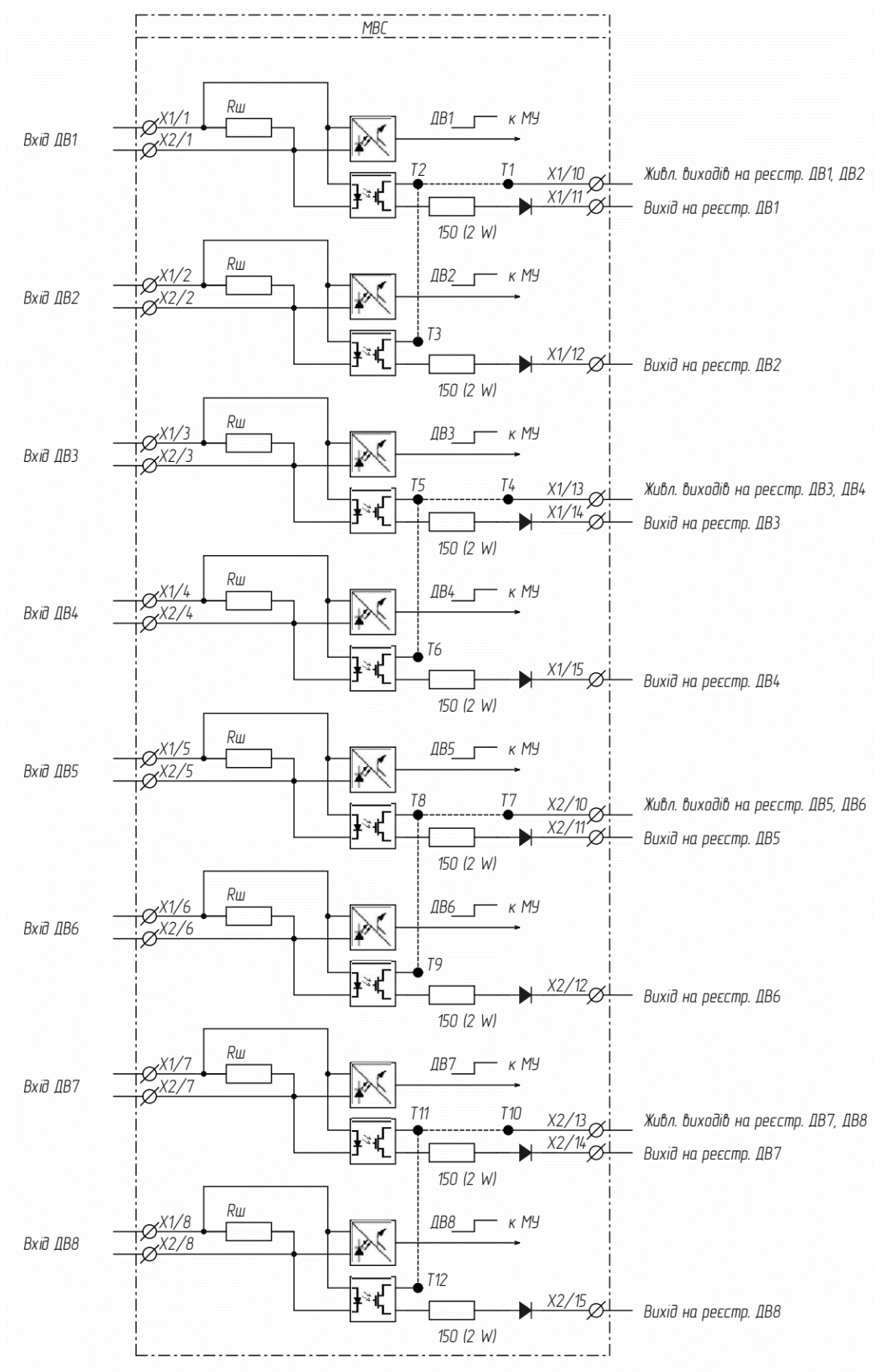
Рисунок 6.1.2.3 – Модуль MBC (MB-210-Zx.0812(I), MB-210-Zx.0722(I))
