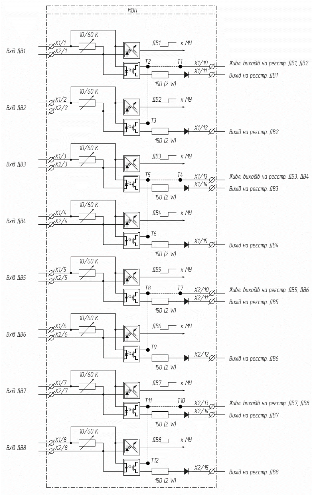
Рисунок 6.1.2.2 – Модуль МВН (МВ-210-Зх.0812(У), МВ-210-Зх.0722(У))
