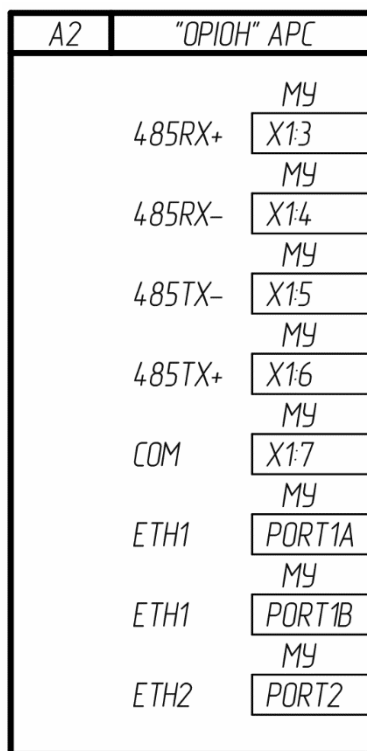
Рисунок 10.6.2.2 – Інтерфейси (виконання APC «ІЕС 61850»)
