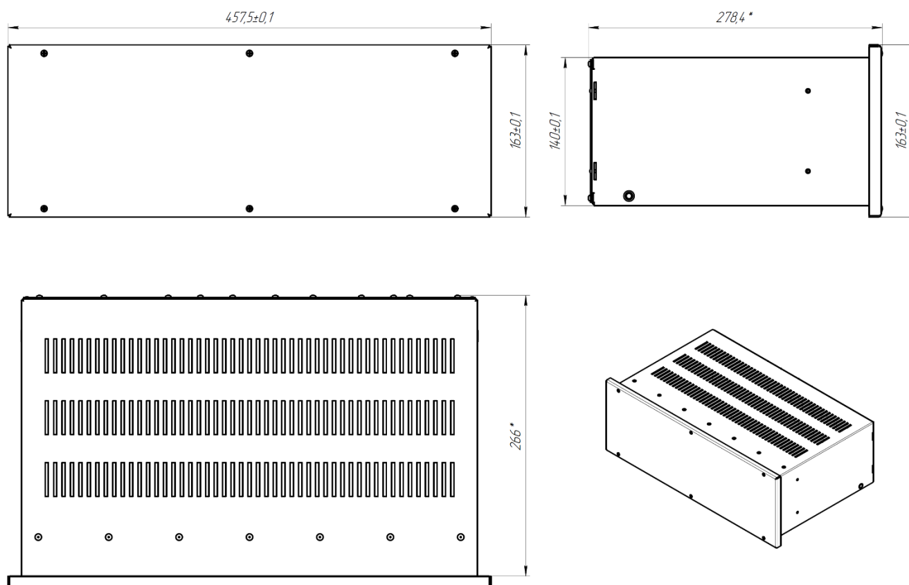
Рисунок 3.1 - Габаритні розміри (APC A)
