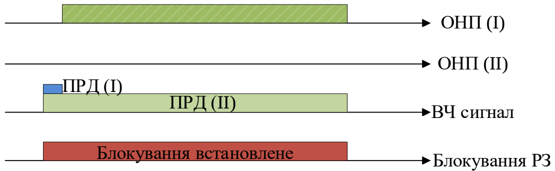
Рисунок 8.1.2.1 - КЗ на "суміжний" ПЛ
