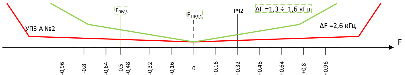
Два ПРМД «ОРИОН» УПЗА в каналі з ПРМД «ПВЗ (Ива)», «ПВЗ-90М», «АВЗК-80» (використовується функція РЗ, між ПРМД «ОРИОН» УПЗА. Також функція КА) «ОРИОН» УПЗА (№1), «ОРИОН» УПЗА (№2), «ПВЗ» (№3)
