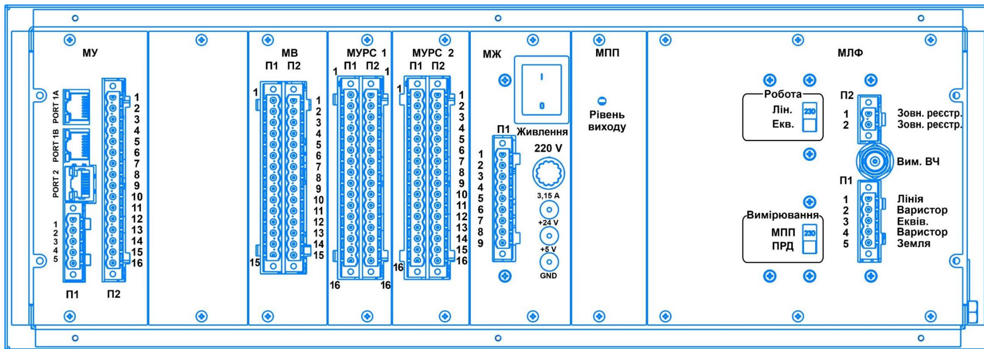
Рисунок 4.4 – Зовнішній вигляд «ОΡΙΟΝ» УПЗА зі сторони підключення
