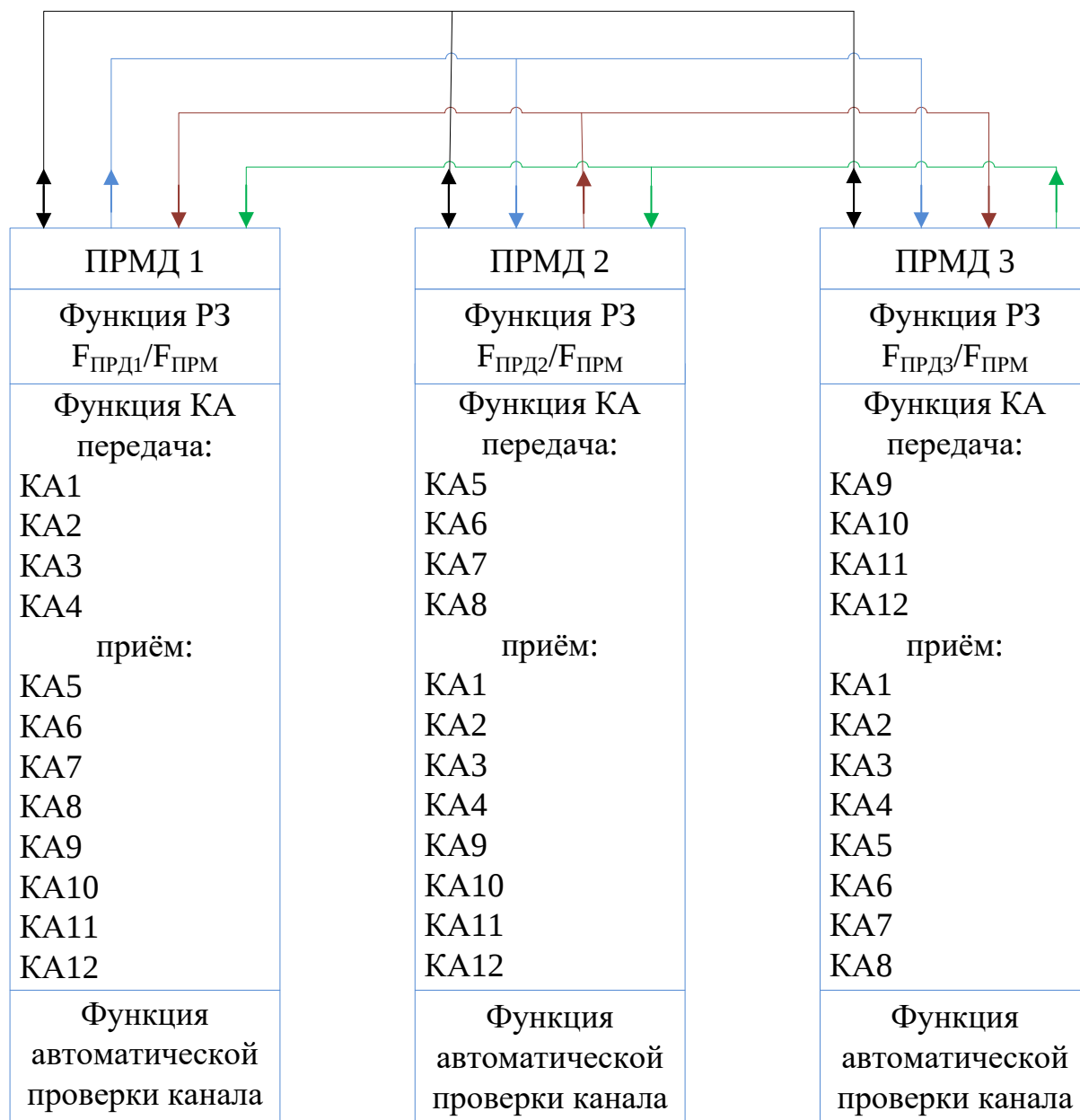
Рисунок 8.4.3 - ВЧ канал з трьома ПРМД «ОПІОН» УПЗА
