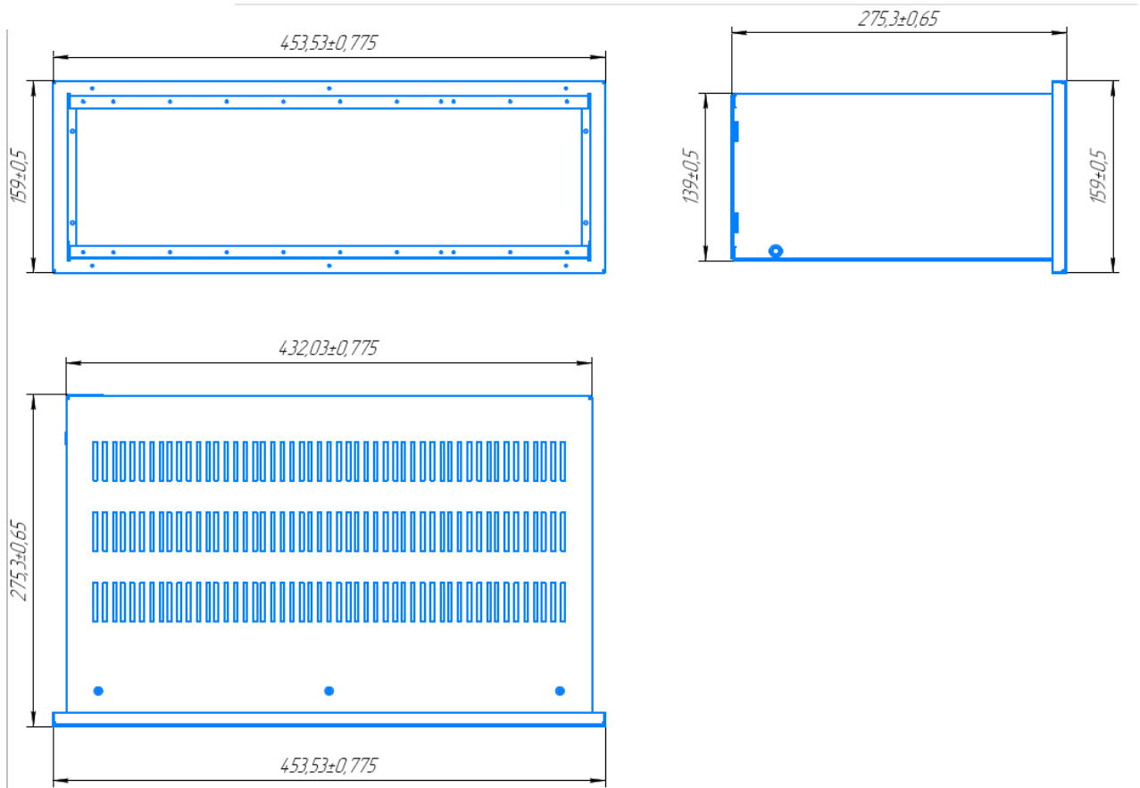
Рисунок 4.1 - Габаритні розміри
