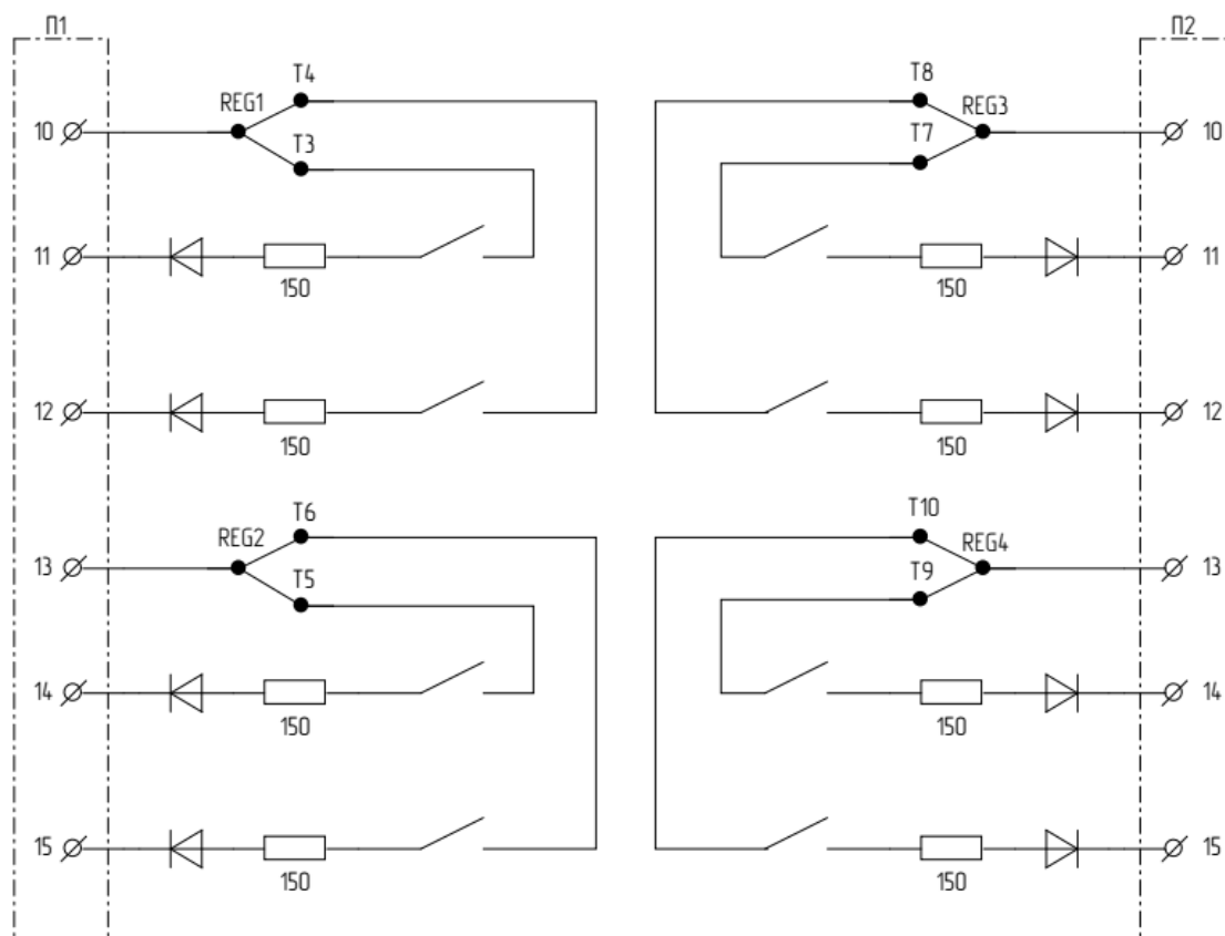
Рисунок 9.3.2 – Схема вихідних кіл модуля MB
