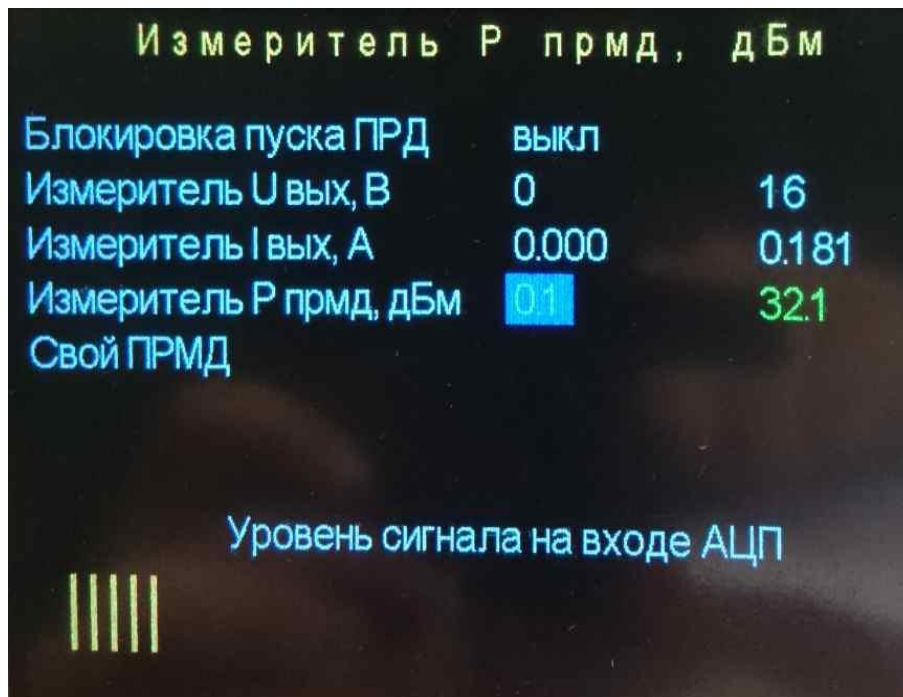
Рисунок 11.9.2.1 – Калибровка вимірювача Упрмд «свій»
