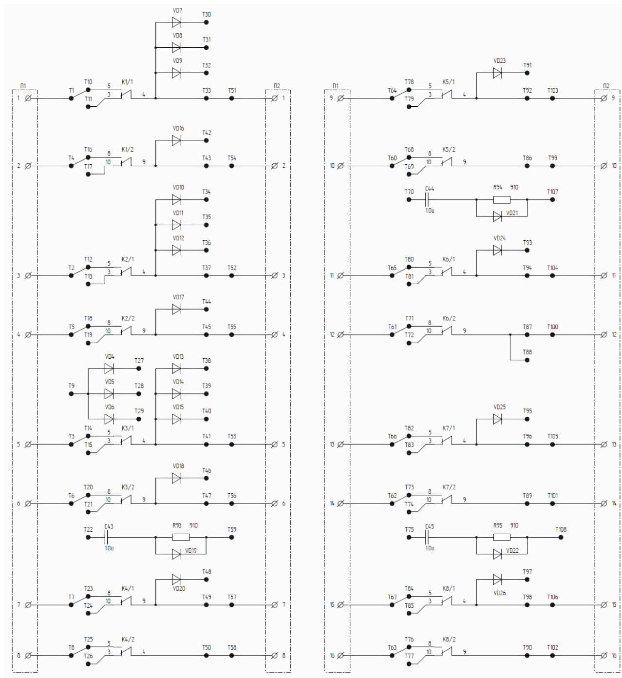
Рисунок 9.2.2 – Схема вихідних реле модуля МУРС 2
