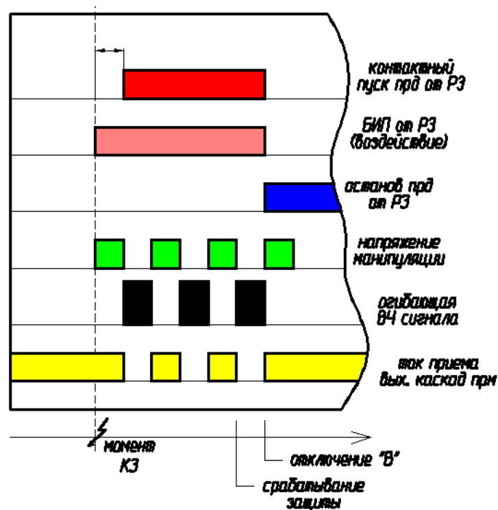
Рисунок 11.13.1 - Приблизний вид осцилограми при КЗ на ПЛ, що захищається
