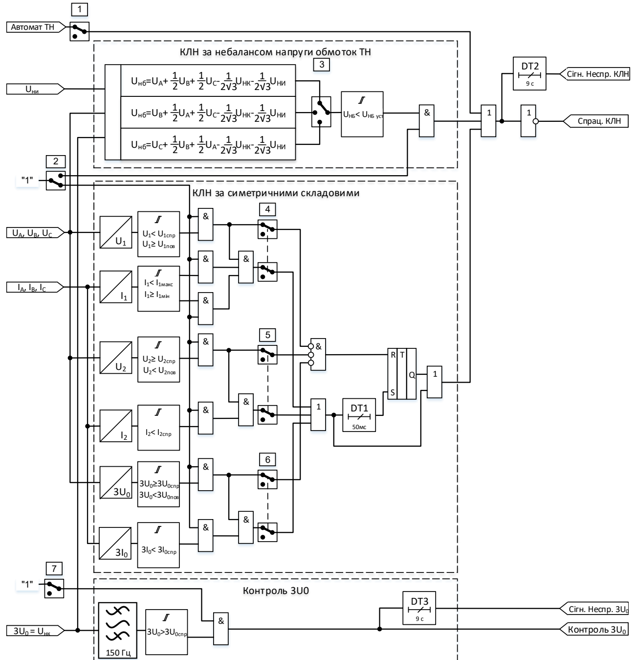
Рисунок 4.9.1 – Схема контролю ланцюгів напруги
