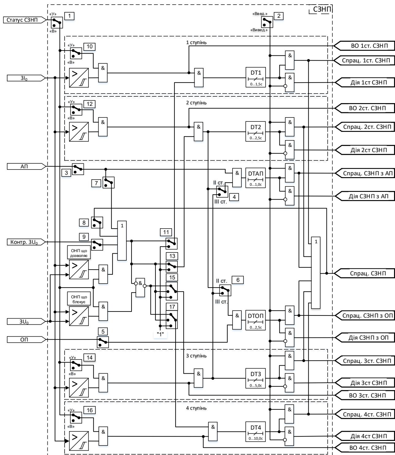
Рисунок 4.1.3.1 Схема СЗНП
