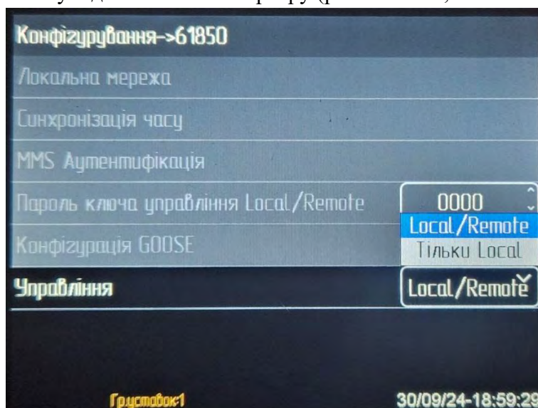
Рисунок 5.4.18.1. Меню «Налаштування 61850»
