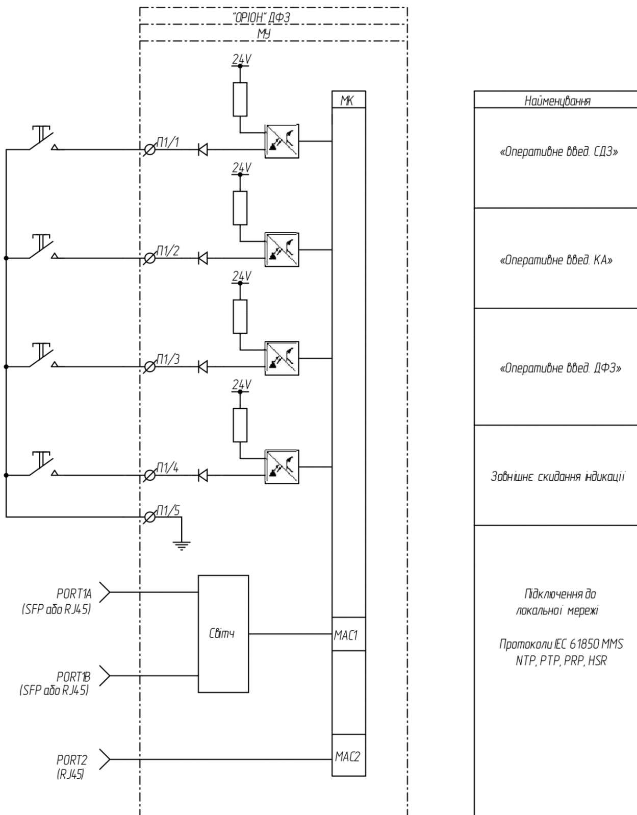
Рисунок 14.5.1 Схема підключення до модуля МУ
