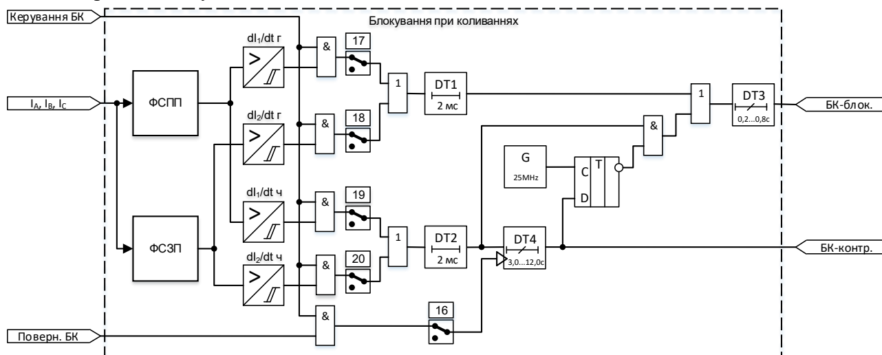
Рисунок 4.1.2.3 Схема БК
