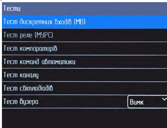
Рисунок 5.6.1.1 – Тести
