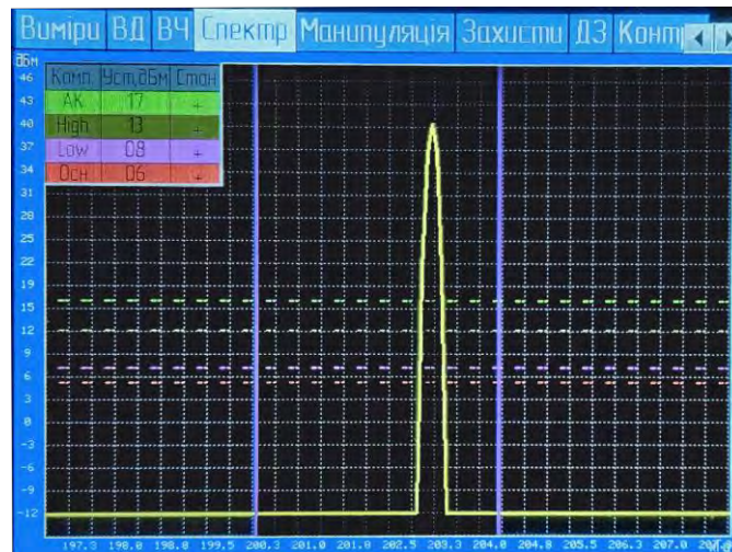
Рисунок 5.8.4 – Вкладка «Спектр».
