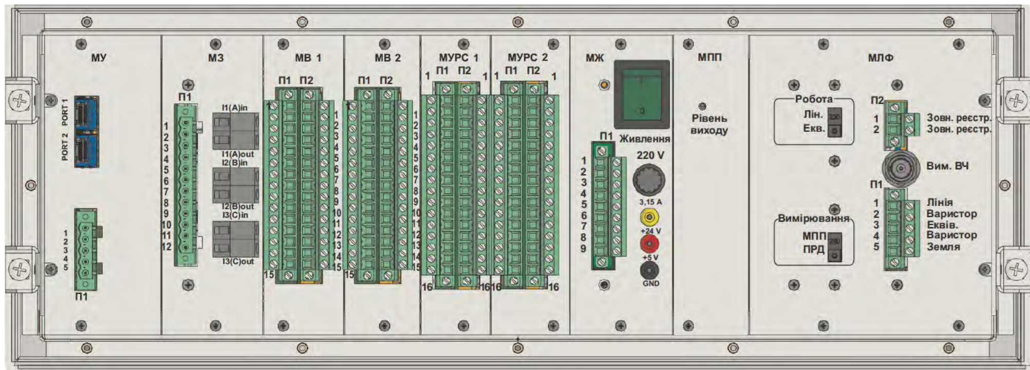
Рисунок 6.6 – Зовнішній вигляд «ОΡΙΟΝ» ДФЗ зі сторони підключення (виробництво після 01.10.2025)
