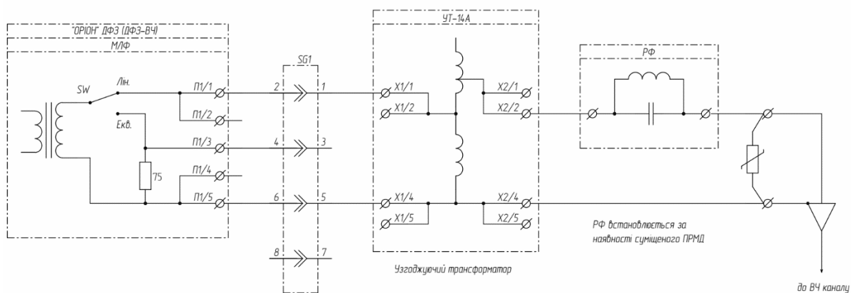
Рисунок 14.6.1 Схема підключення до ВЧ каналу
