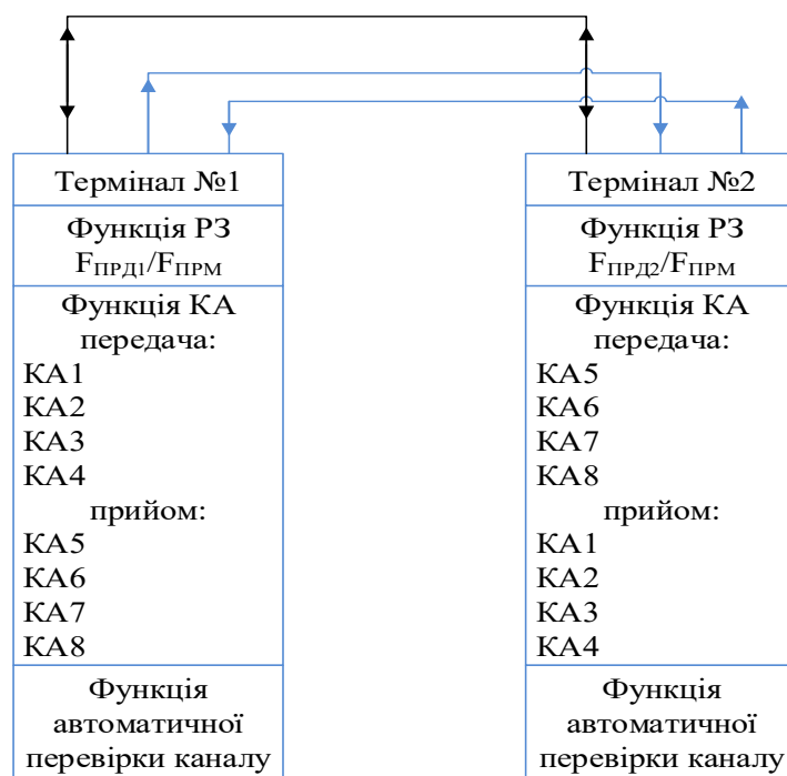
Рисунок 4.4.2 - ВЧ канал с двома терміналами «ОРИОН» ДФЗ
