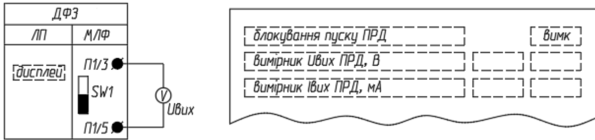
Рисунок 5.4.14.2 – Калібрування передавача
