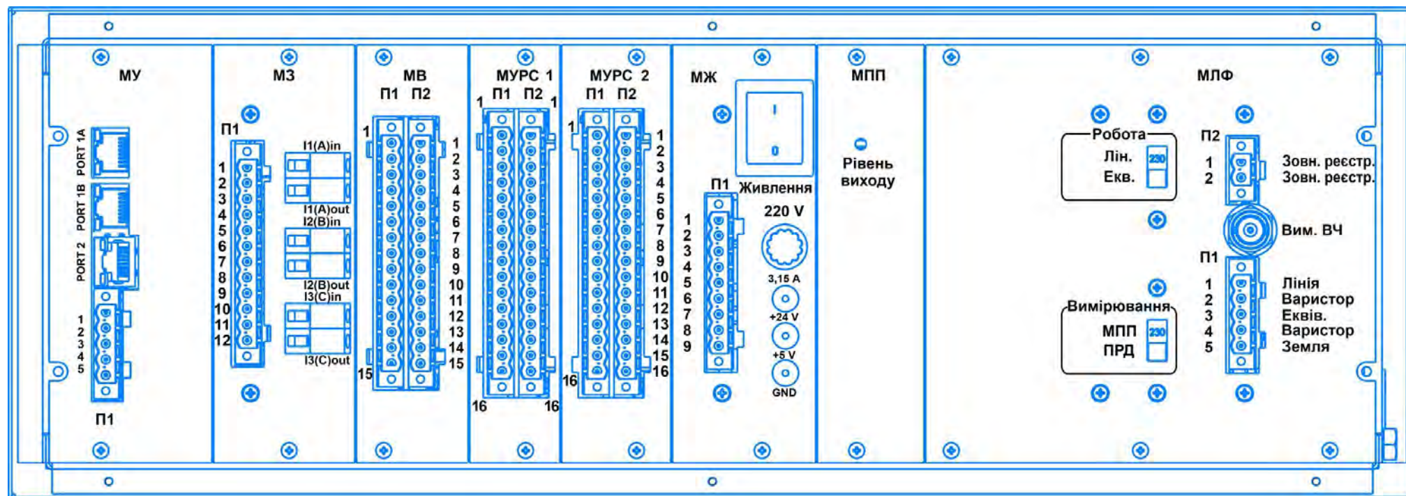
Рисунок 6.5 – Зовнішній вигляд «ОΡΙΟΝ» ДФЗ зі сторони підключення (виробництво до 01.10.2025)
