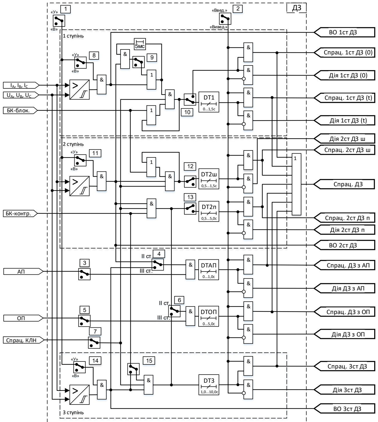
Рисунок 4.1.2.2 Схема дистанційного захисту
