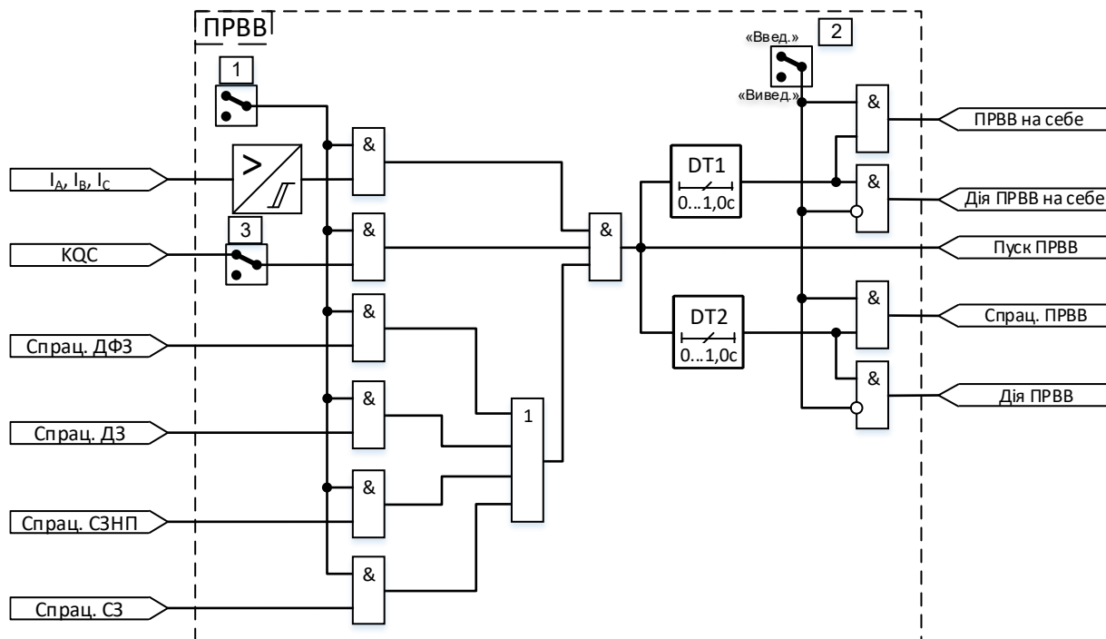
Рисунок 4.2.1 – Схема ПРВВ
