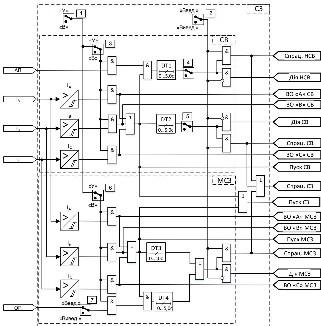
Рис. 4.1.4.1 Схема СЗ
