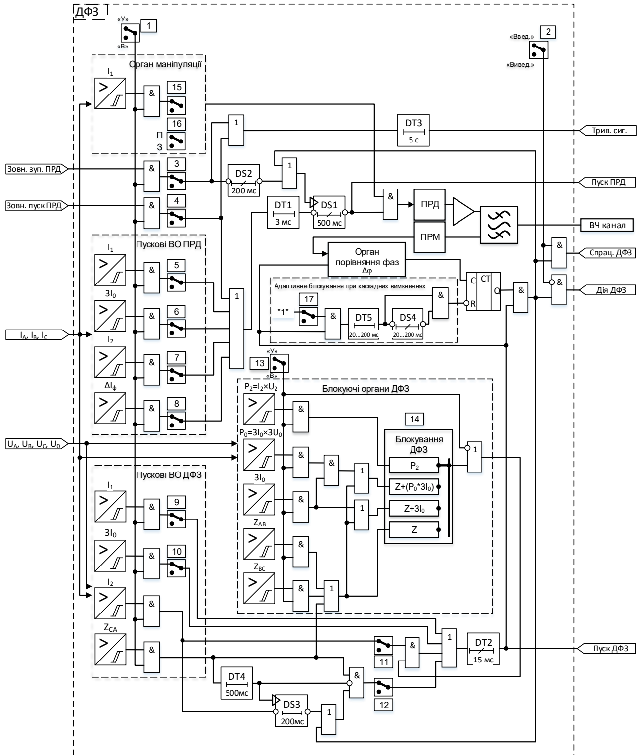
Рисунок 4.1.1.3 Схема ДФЗ
