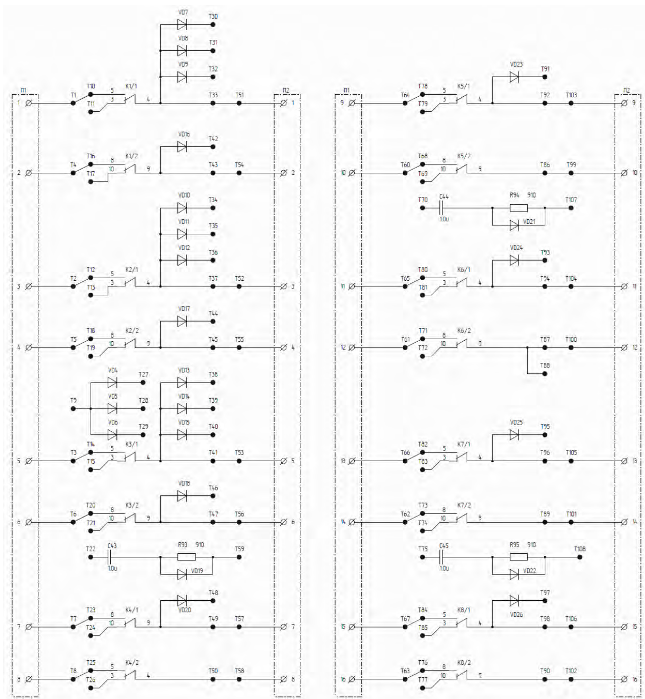
Рисунок 14.3.1.2 – Схема вихідних ланцюгів модуля МУРС2
