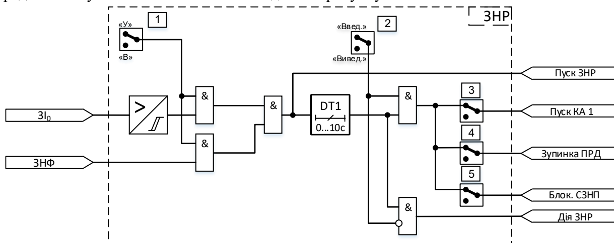
Рисунок 4.3.1 – Схема ЗНР
