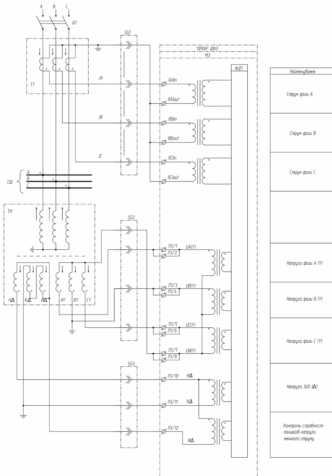
Рисунок 14.4.1 Схема підключення ланцюгів струму та напруги
