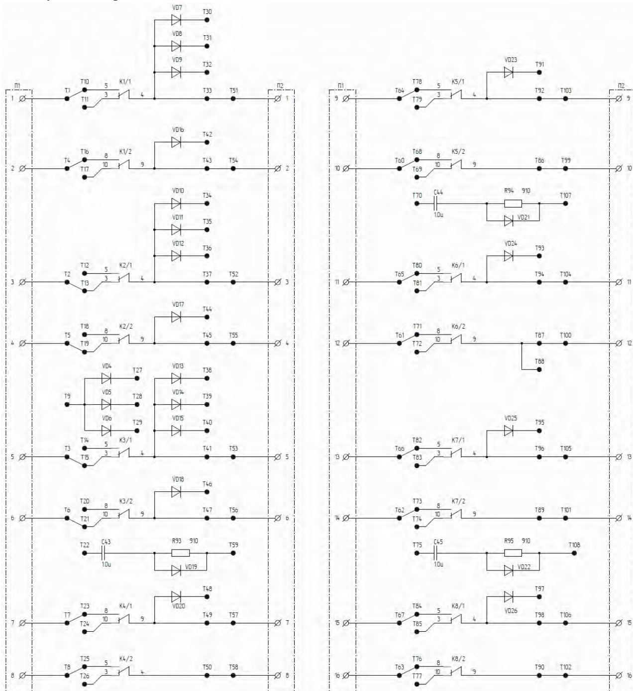
Рисунок 14.3.1.1 – Схема вихідних ланцюгів модуля МУРС1
