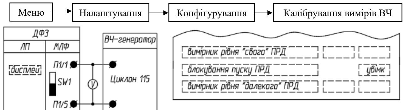
Рисунок 5.4.14.3 – Калібрування приймача
