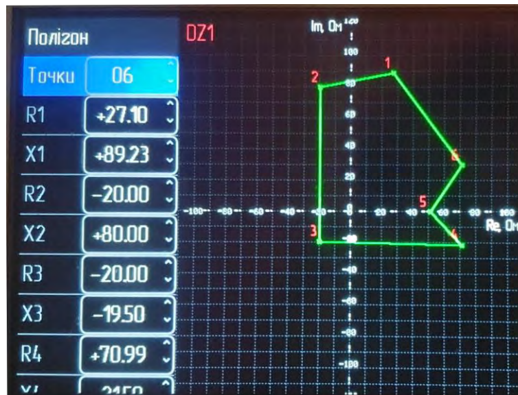
Рисунок 5.4.6.3 – Задання точок полігональної характеристики
