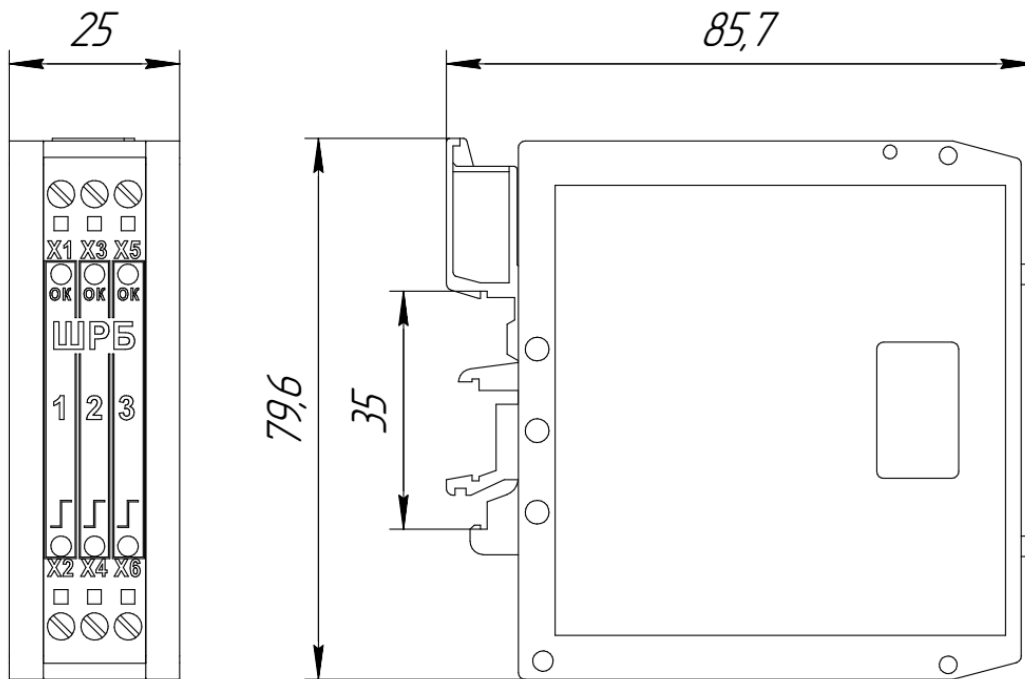
Рисунок 4.1 - Габаритный чертеж ШРБ-17
