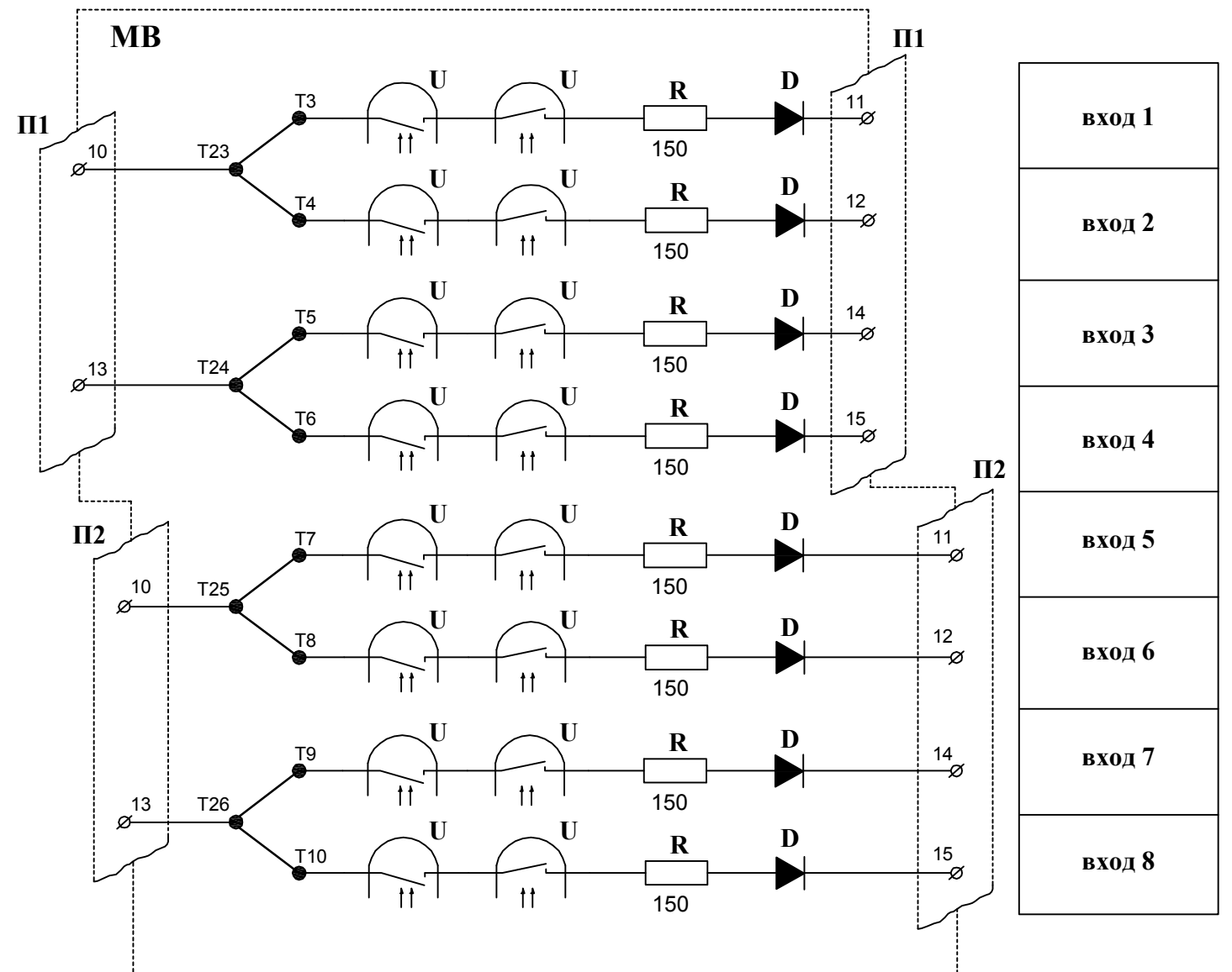
Рисунок 10.4 - Аппаратное конфигурирование цепей регистрации МВ "по умолчанию"
