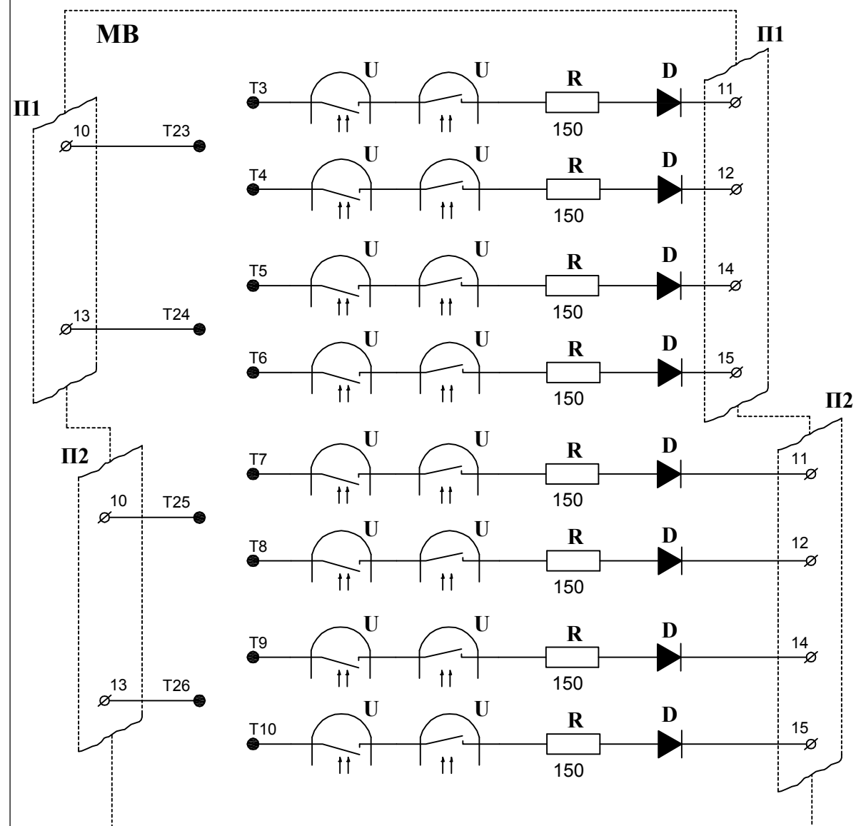
Рисунок 10.3 - Цепи выхода на внешний регистратор модуля дискретных входов
