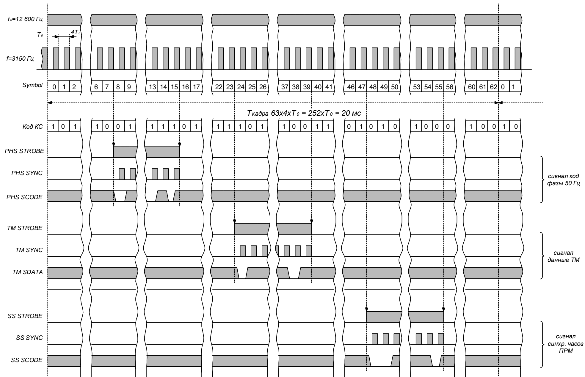
Рисунок 7.5 - Временная диаграмма формирования контрольного сигнала КС с наложением информации синхронизации часов, данных ТМ и кода фазы промышленной частоты
