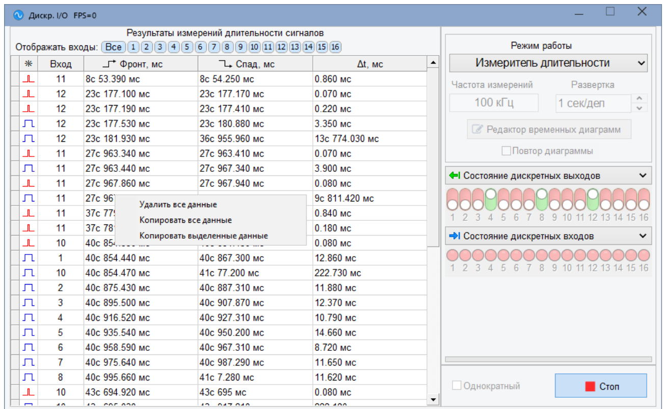
Рисунок 10.11.3.1 – Внешний вид панели «Дискр. I/O» в режиме работы «Измеритель длительности»
