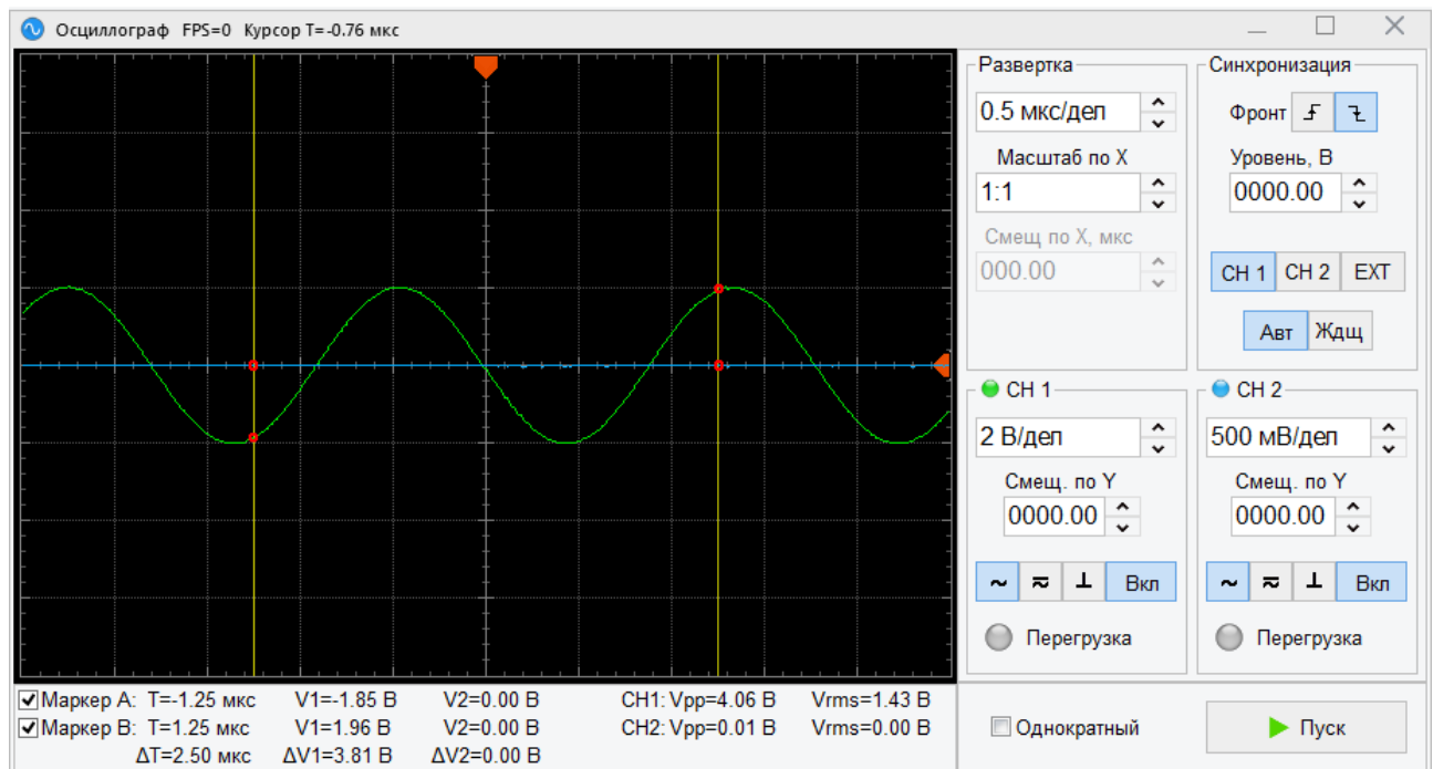
Рисунок 10.2.2.1 – Внешний вид панели осциллографа
