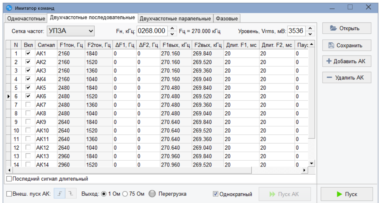
Рисунок 10.8.4.1 – Внешний вид панели имитатора команд «Двухчастотные последовательные»
