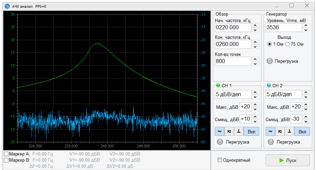
Рисунок 10.4.2.1 – Внешний вид панели измерителя АЧХ
