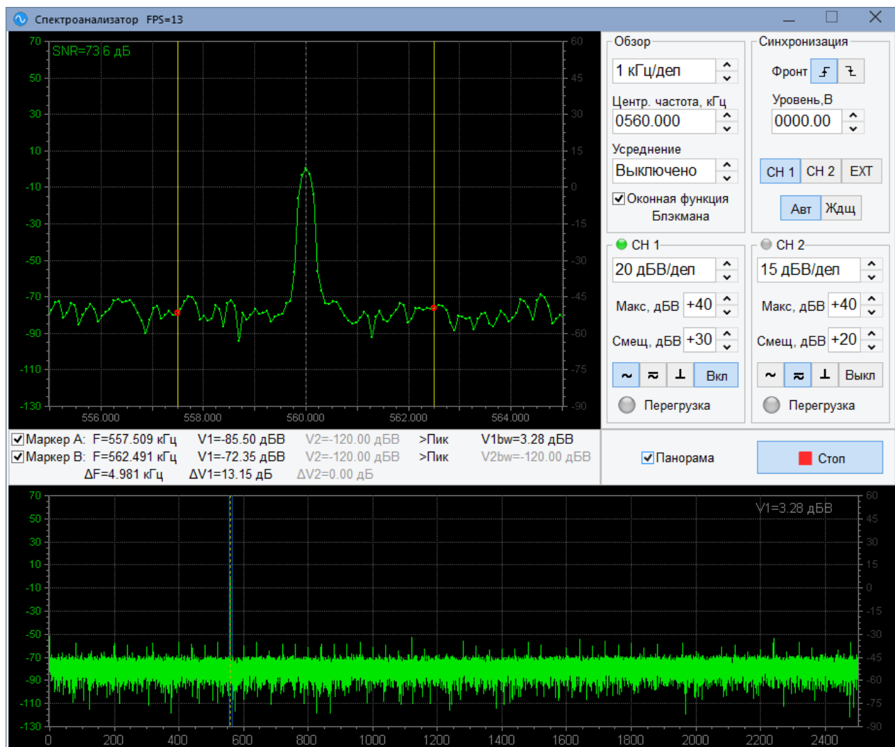
Рисунок 10.3.2.2 – Внешний вид панели спектроанализатора в режиме «Панорама»
