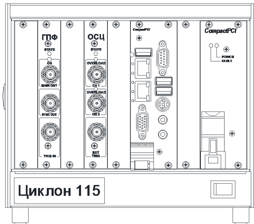
Рисунок 4.1.1 – Внешний вид прибора (Модификация 1)
