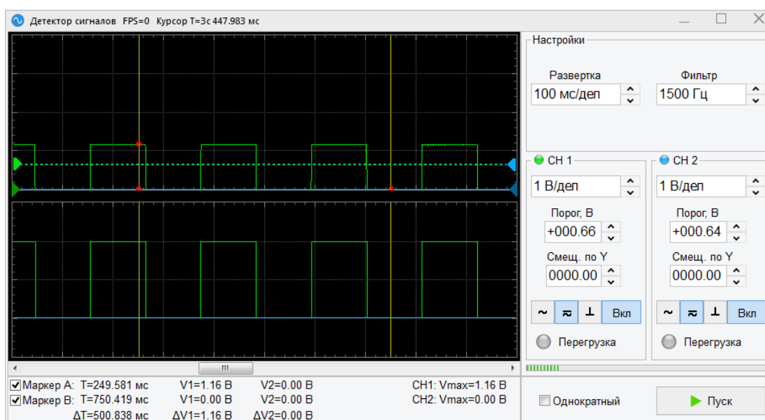
Рисунок 10.10.2.1 – Внешний вид панели детектора сигналов
