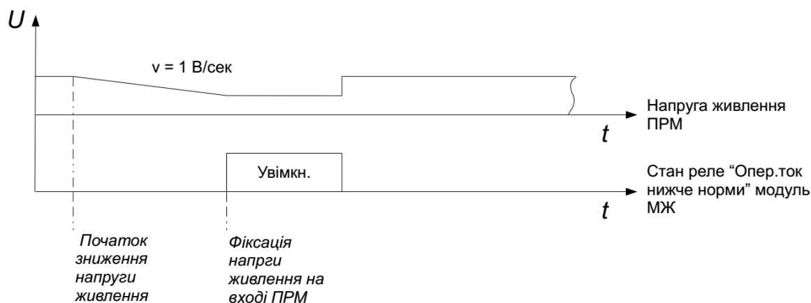
Рисунок 8.15.2 – Часова діаграма перевірки сигнал. «Опер.струм нижче норми»
