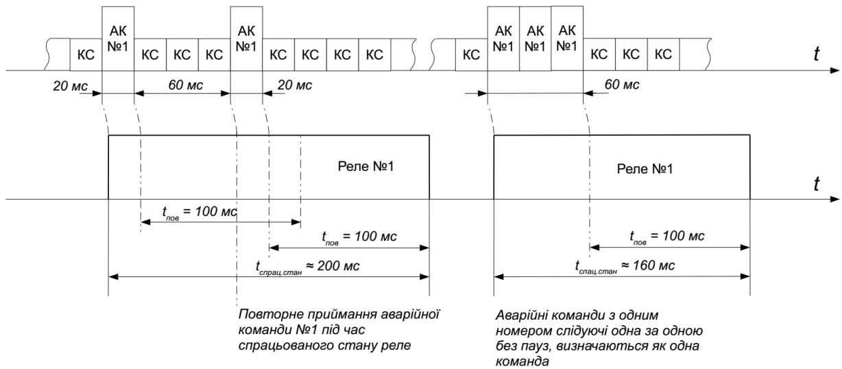
Рисунок 5.2.3.3 - Приймання аварійної команди з різною тривалістю
