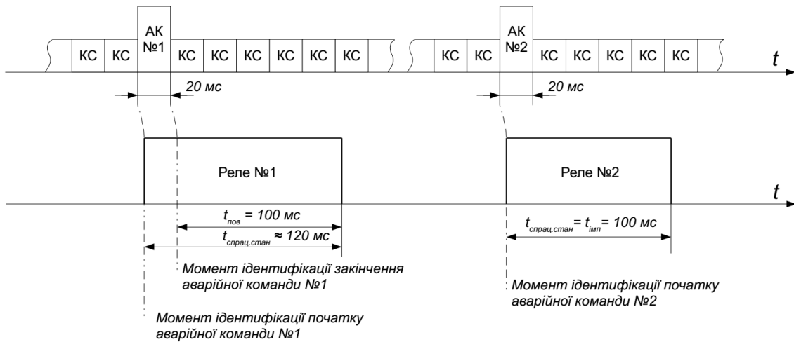
Рисуюнок 5.2.3.1 - Приймання двох аварійних команд
