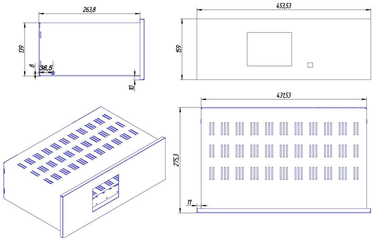
Рисунок 3.1 – Стандартний корпус «ОΡΙΟΝ» ΑΠΚ RХ
