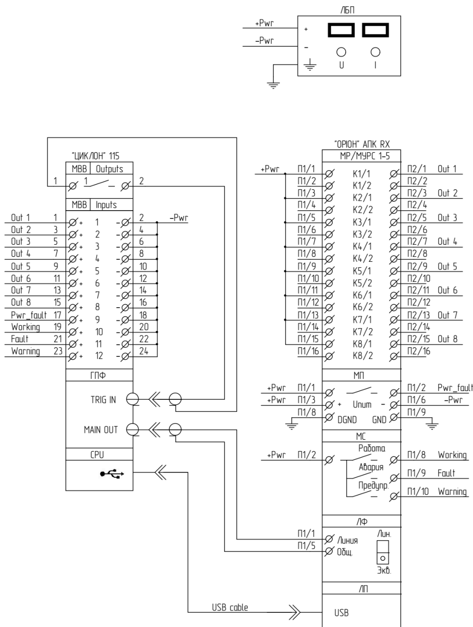
Рисунок 8.12.3 – Електрична схема з'єднання з використанням «ЦИКЛОН» 115
