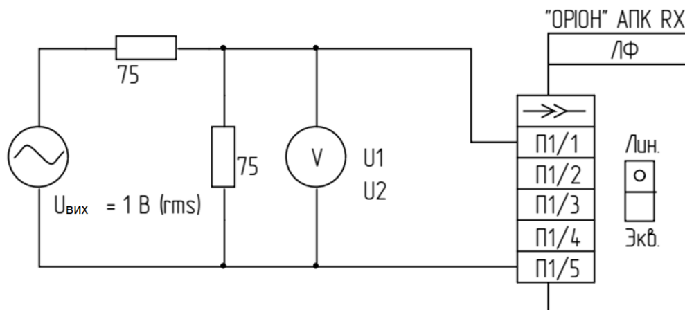
Рисунок 8.9.1 – Електрична схема вимірювань
