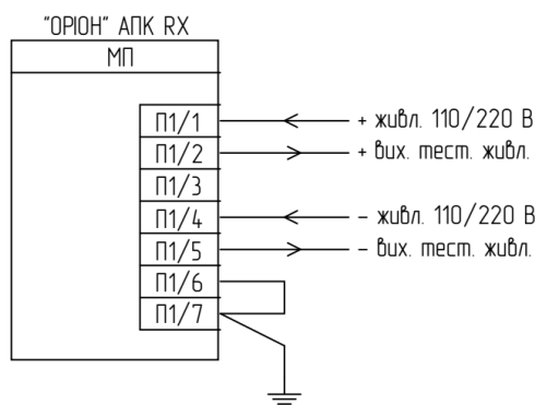
Рисунок 6.4.1.1 – Схема підключення МЖ («П1» 7 контактів)
