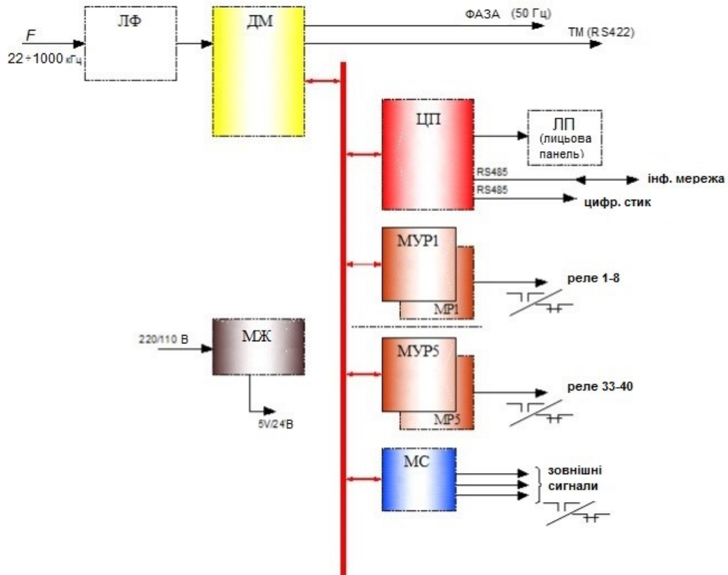
Рисунок 5.5.1 - Структурна схема «ОРИОН» АПК RX
