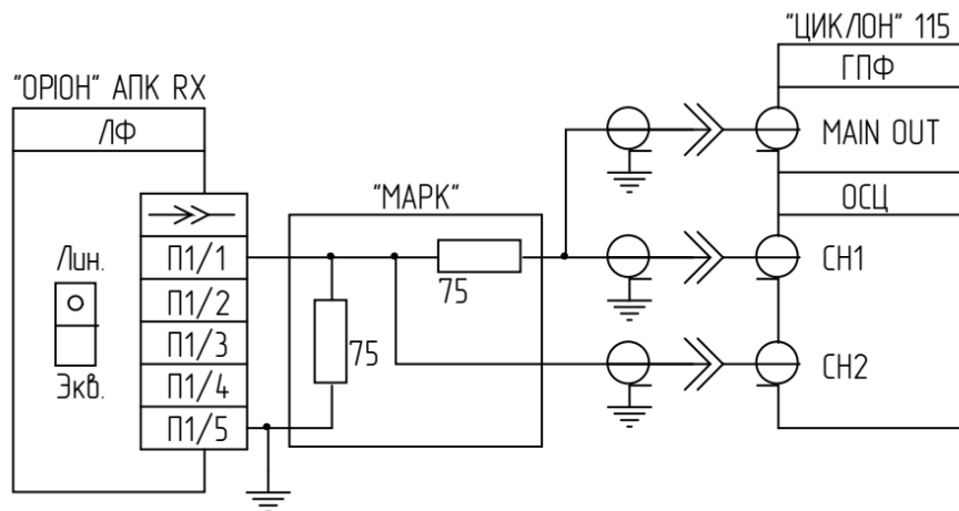
Рисунок 8.9.2 – Схема підключення
