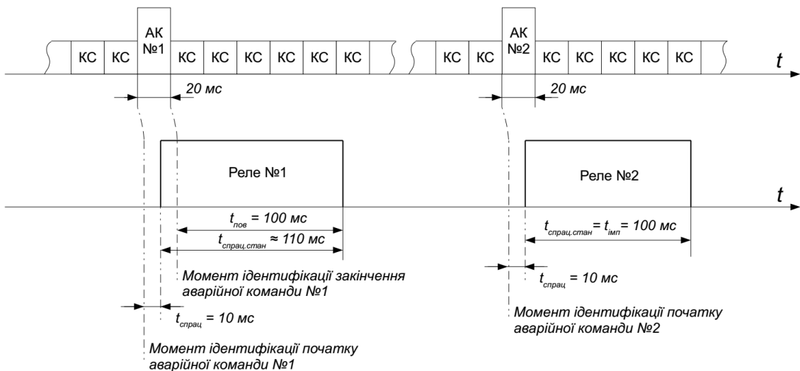
Рисуюнок 5.2.3.2 - Приймання двох аварійних команд з затримкою на спрацювання
