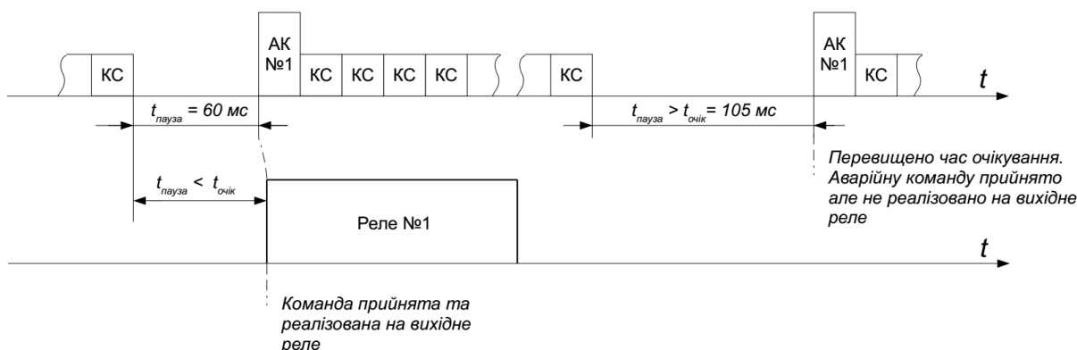
Рисунок 5.2.3.6 - Відсутність приймання контрольного сигналу в умовах інтенсивних комутаційних завд
